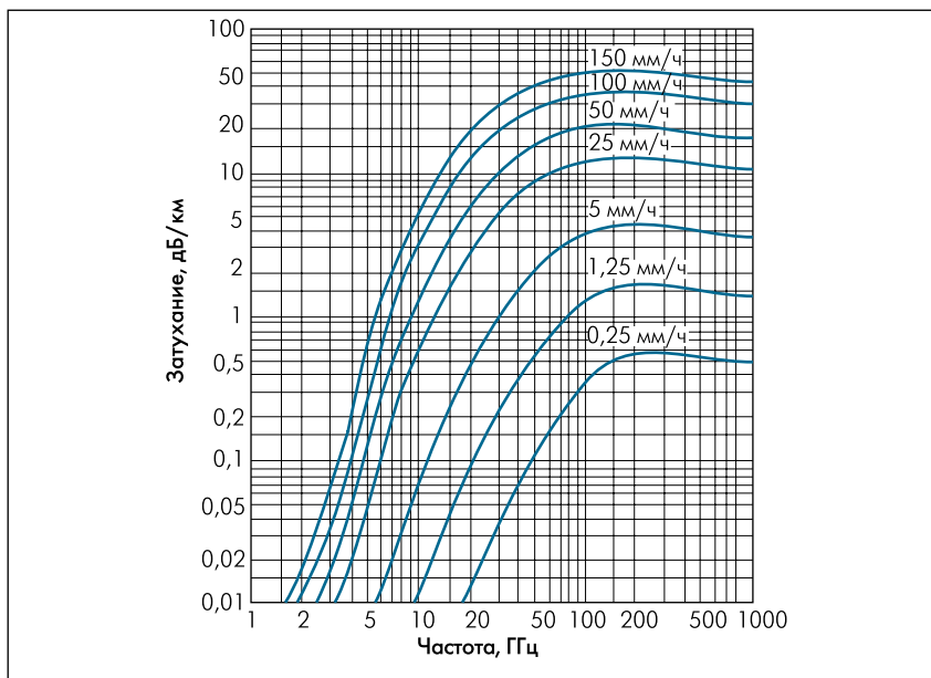
Рис.2. Уровень затухания сигнала при осадках
