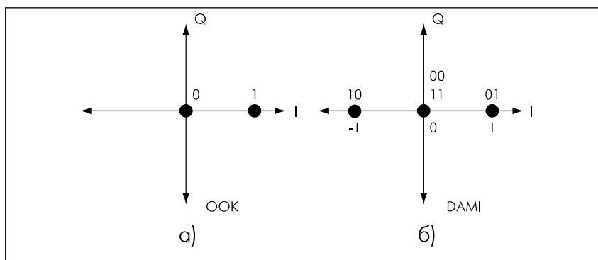
Рис.7. Сигнальные созвездия при модуляции OOK (а) и DAMI (б)
