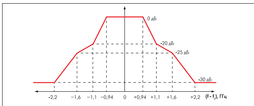
Рис.6. Спектральная маска канала при передаче в стандарте 802.15.3с
