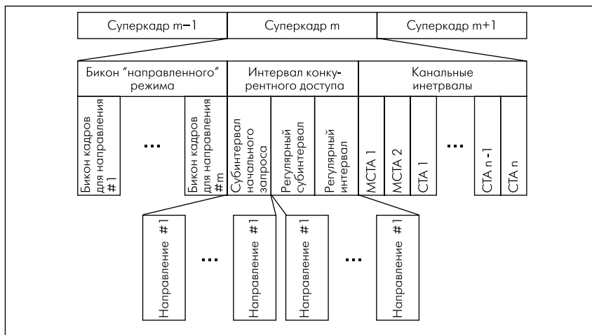
Рис.5. Структура суперкадров в квазивсенаправленном режиме стандарта 802.15.3c
