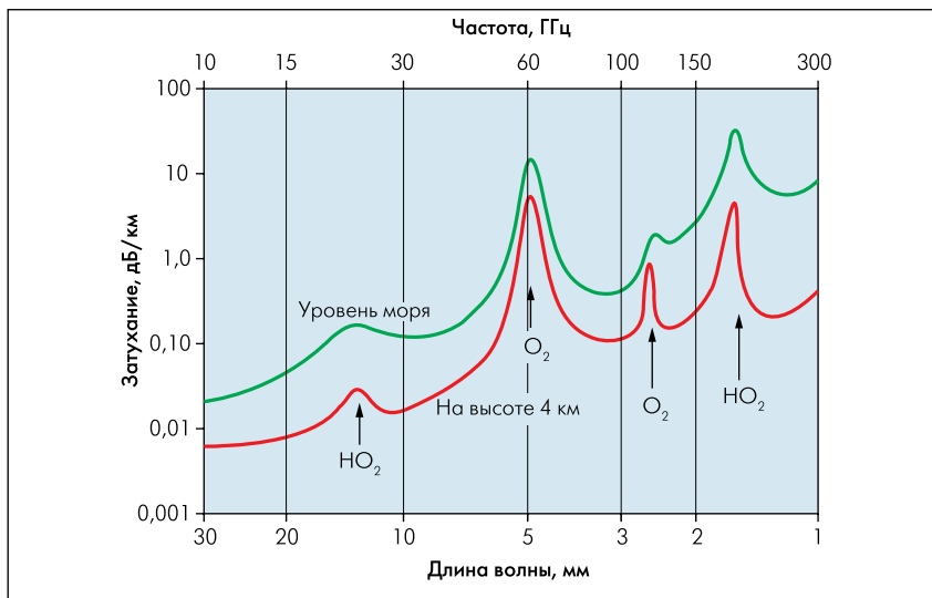
Рис.1. Ослабление сигнала в воздухе за счет атмосферного кислорода и воды (согласно рекомендации ITU-R P.676-5)
